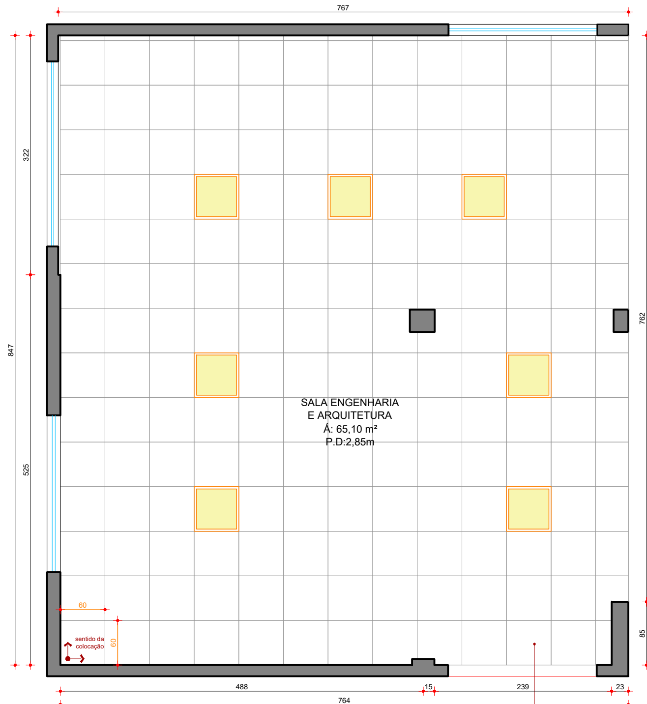
PLANTA DE FORRO Esc.:1/50
