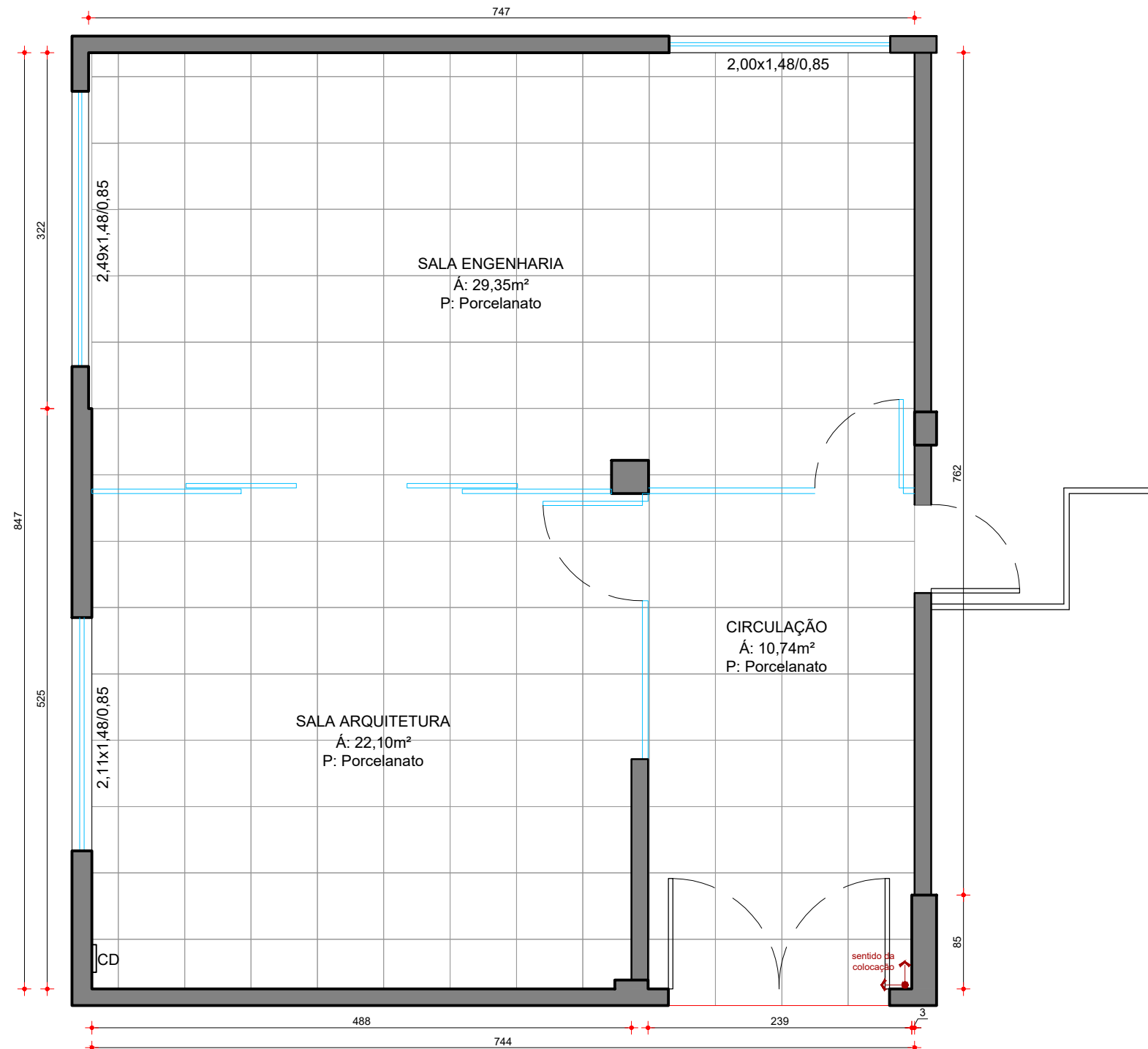
PLANTA BAIXA - PAGINAÇÃO Esc.:1/50
