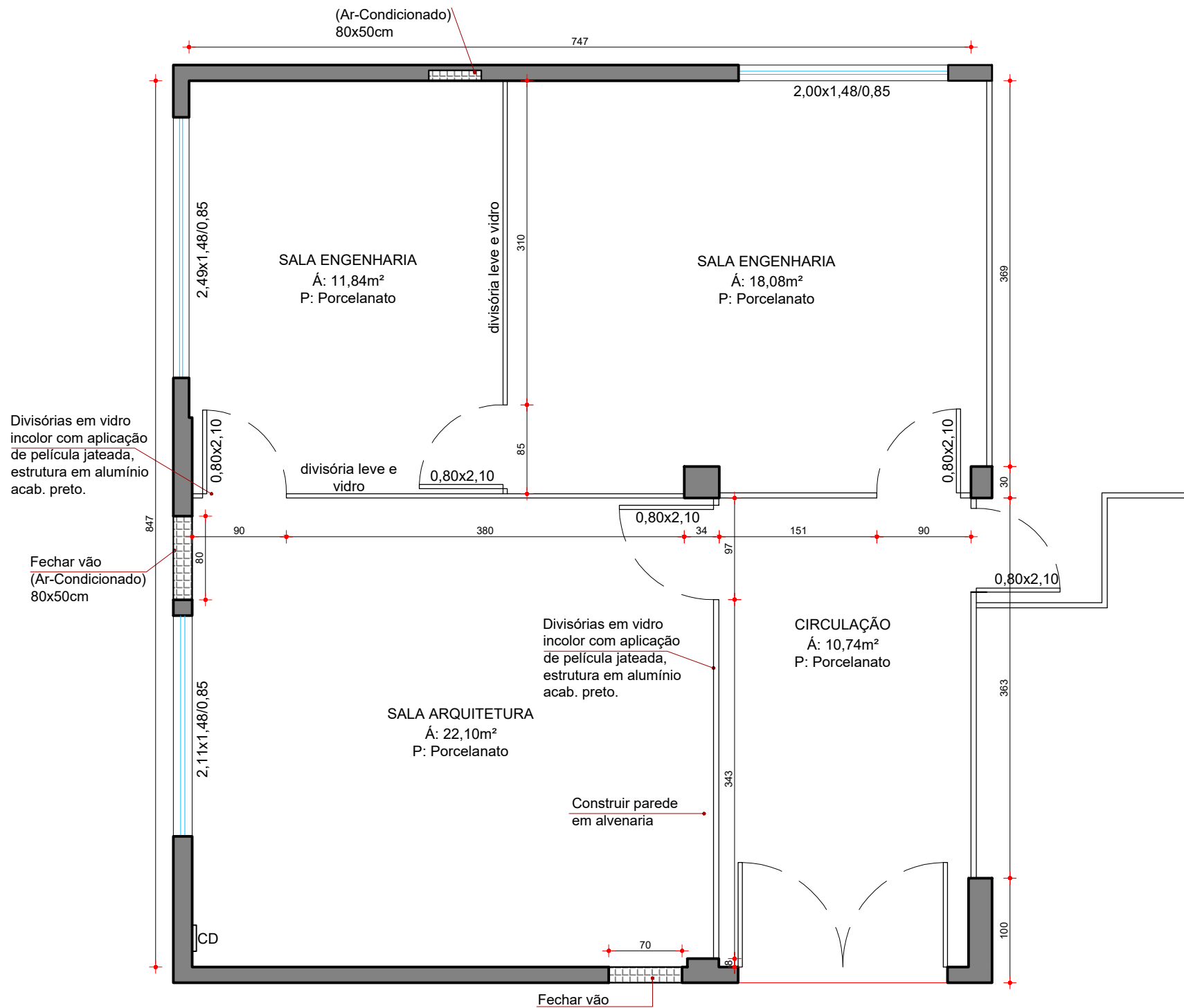
PLANTA BAIXA - CONSTRUIR Esc.:1/50
