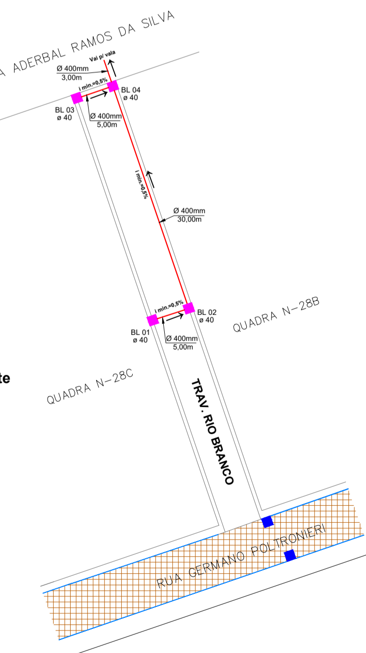
IMPLANTAÇÃO - DRENAGEM PLUVIAL Escala 1/500
