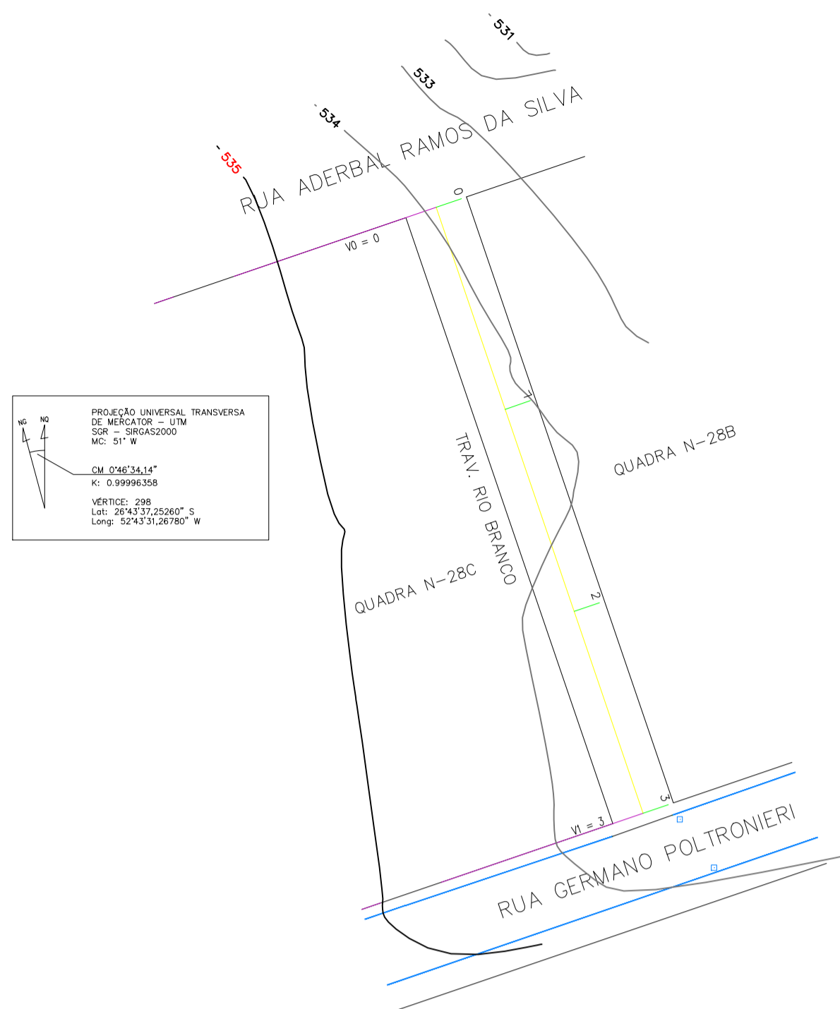
IMPLANTAÇÃO - PLANALTIMÉTRICO Escala 1/1000
