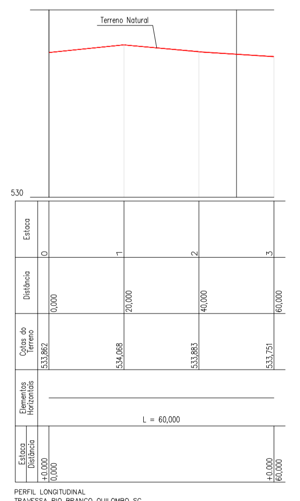
PERFIL LONGITUDINAL TRAVESSA RIO BRANCO QUILOMBO SC ESCALAS H: 1:1000 - V: 1:100
