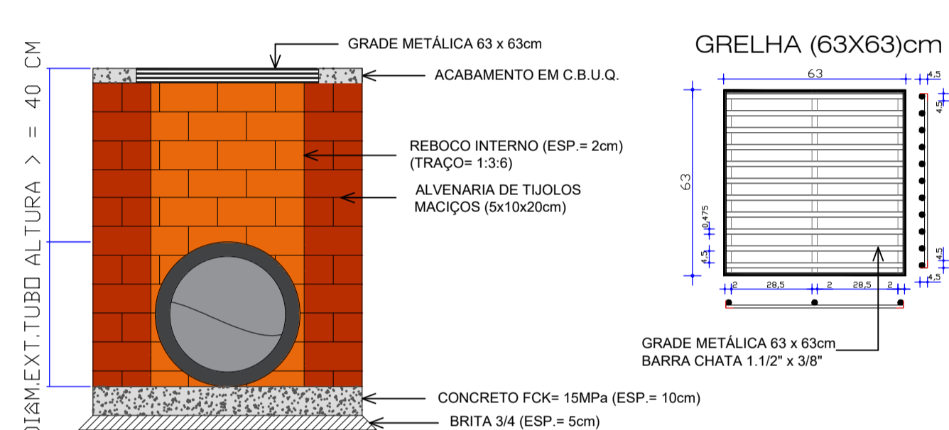
DETALHE 07 -CAIXA COLETORA C/BOCA DE LOBO - TUBO Ø40cm Escala 1:25
