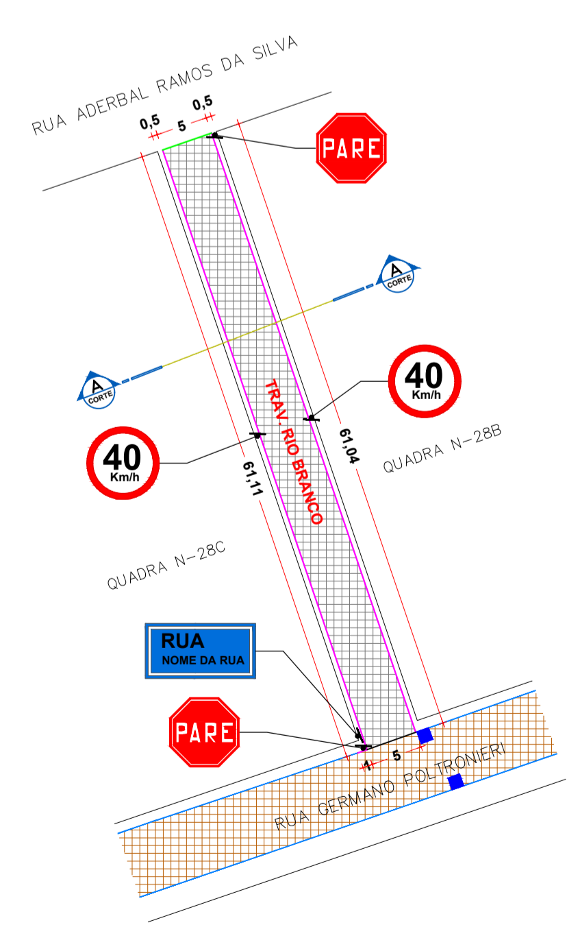
IMPLANTAÇÃO - PLANTA TÉCNICA Escala 1/500 Área = 305,38m 2
