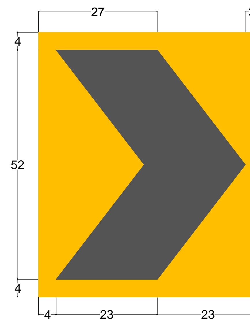
Detalhe - Placa
