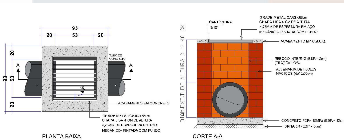
Detalhe 01 – Detalhe Boca de Lobo Ø40cm
