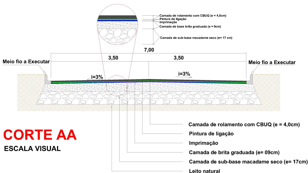
Detalhe 03 – Execução de pavimentação sobre leito natural
