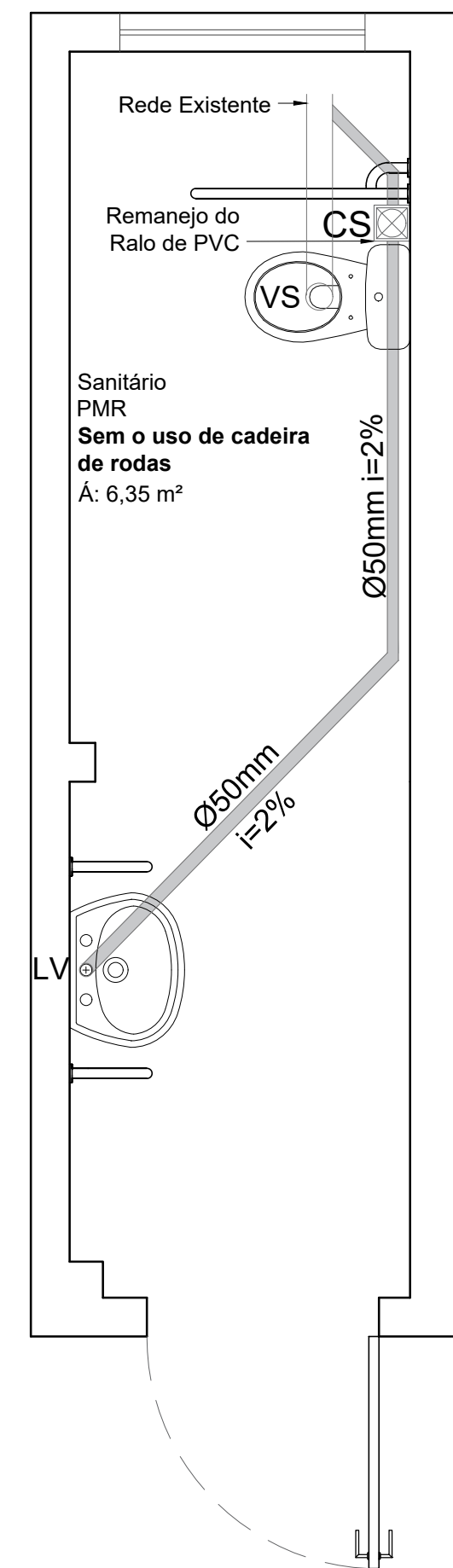
Det. 03 - Planta Baixa Esgoto Escala 1:25
