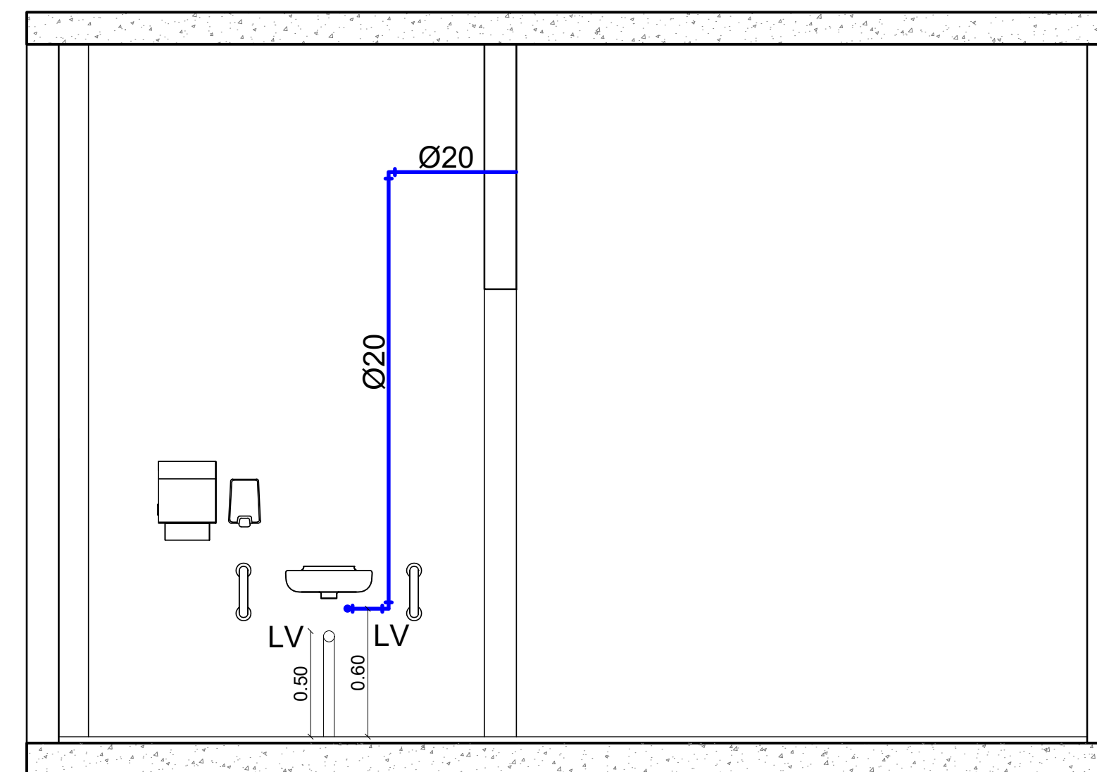
Det. 03 - Vista 02 - Hidrossanitário Escala 1:25
