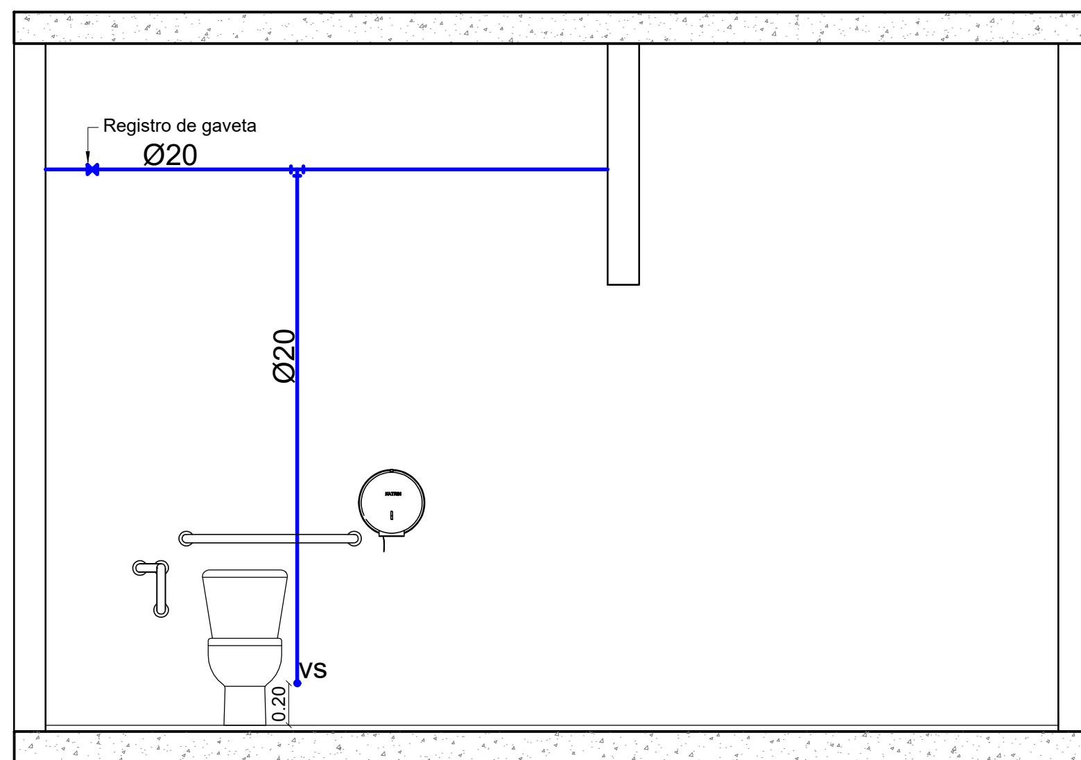
Det. 03 - Vista 01 - Hidrossanitário Escala 1:25
