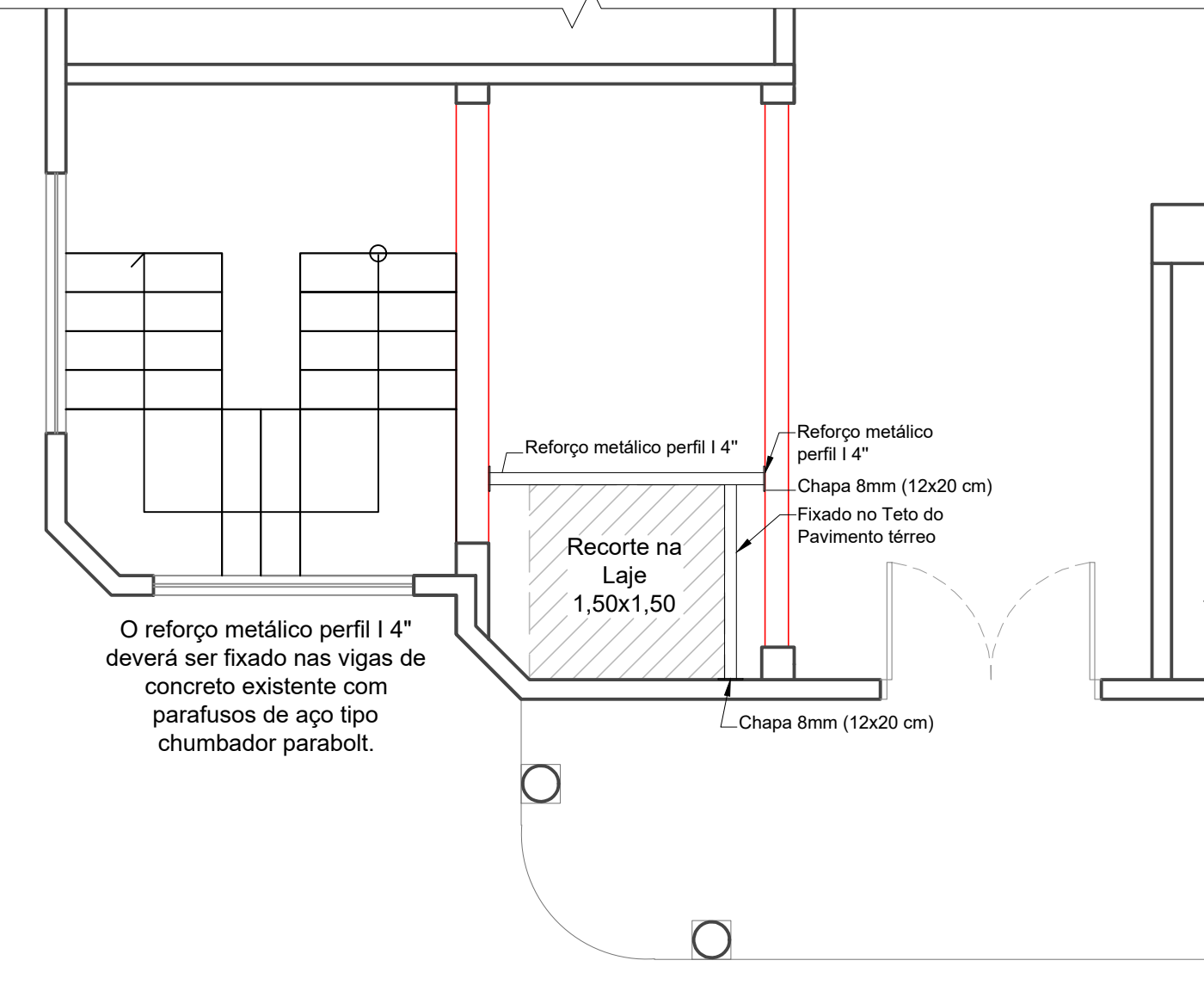
PLANTA BAIXA - TÉRRECO REFORÇO ESTRUTURAL Escala 1:50
