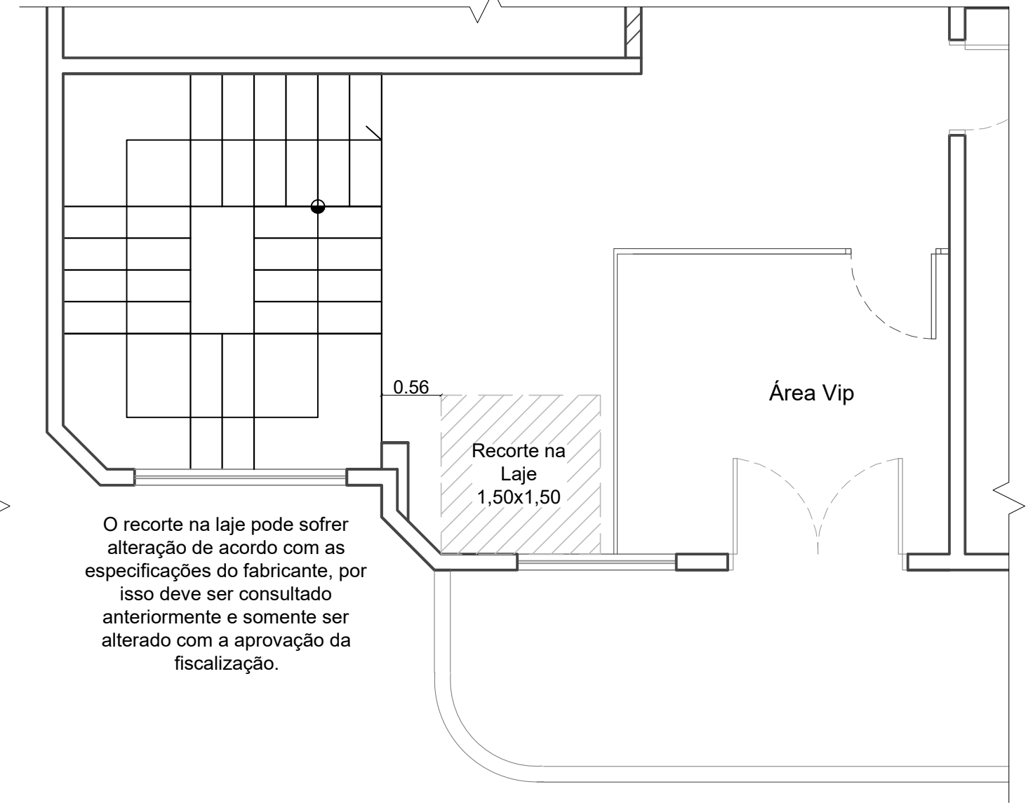
PLANTA BAIXA - RECORTE NA LAJE Escala 1:50
