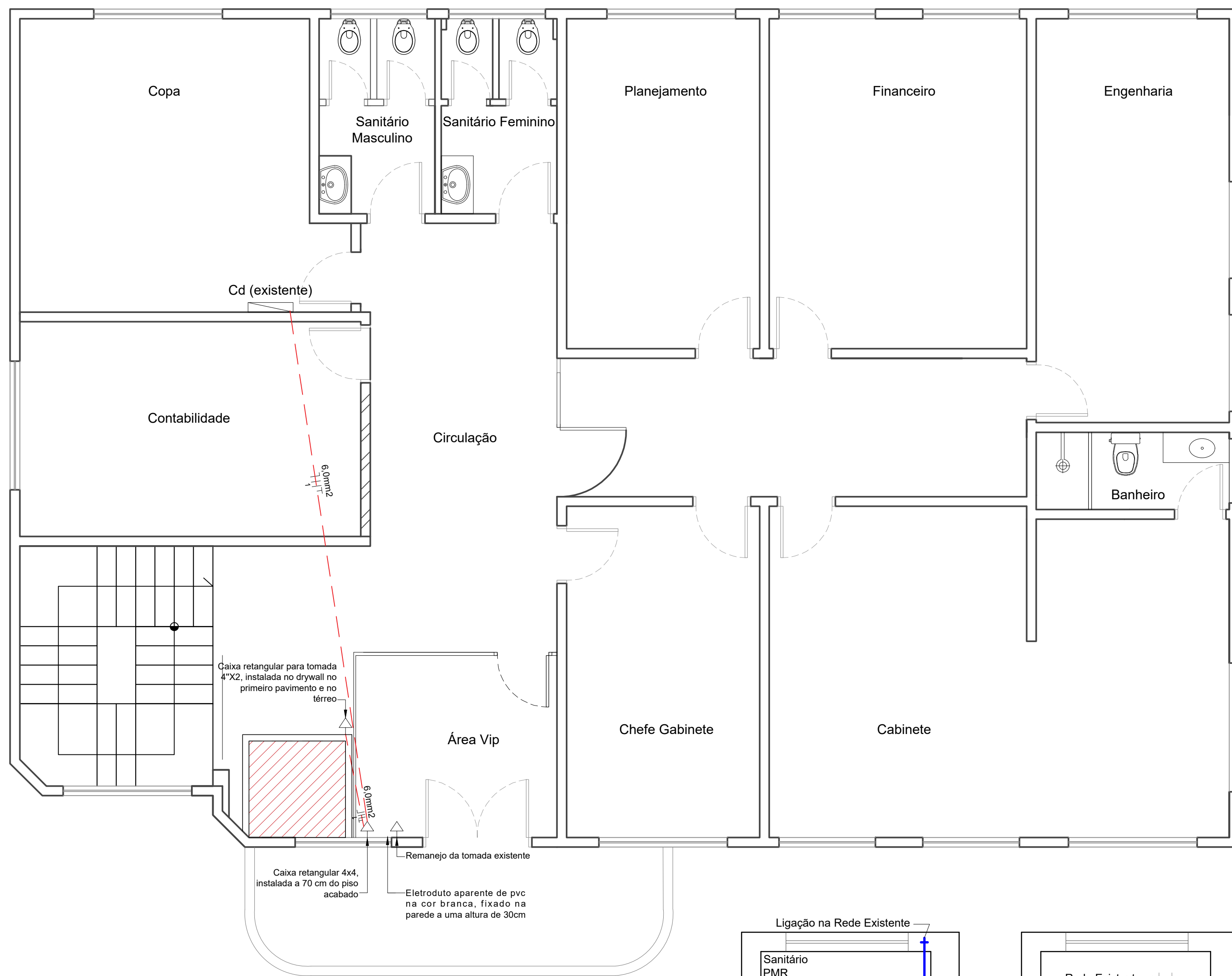
PLANTA BAIXA 1º PAVIMENTO - PROJETO ELÉTRICO Escala 1:50
