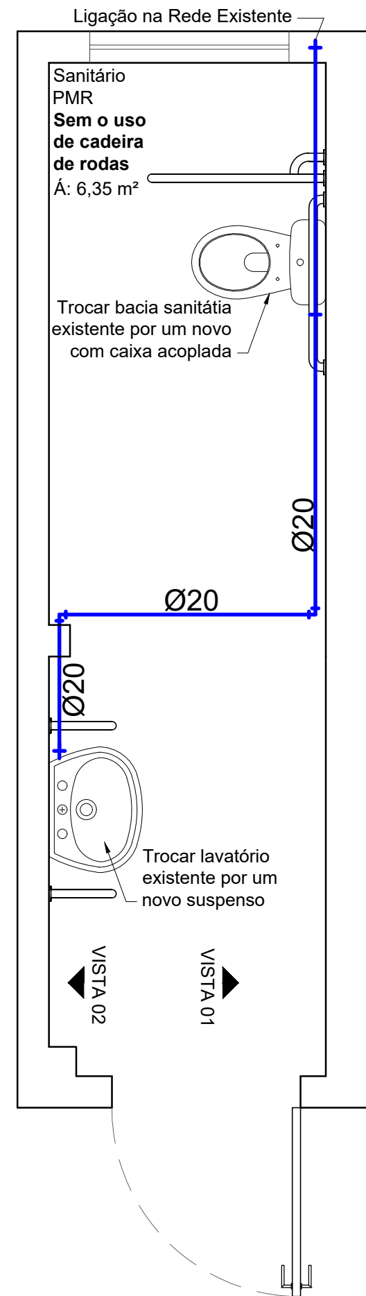
Det. 03 - Planta Baixa Hidráulica Escala 1:25
