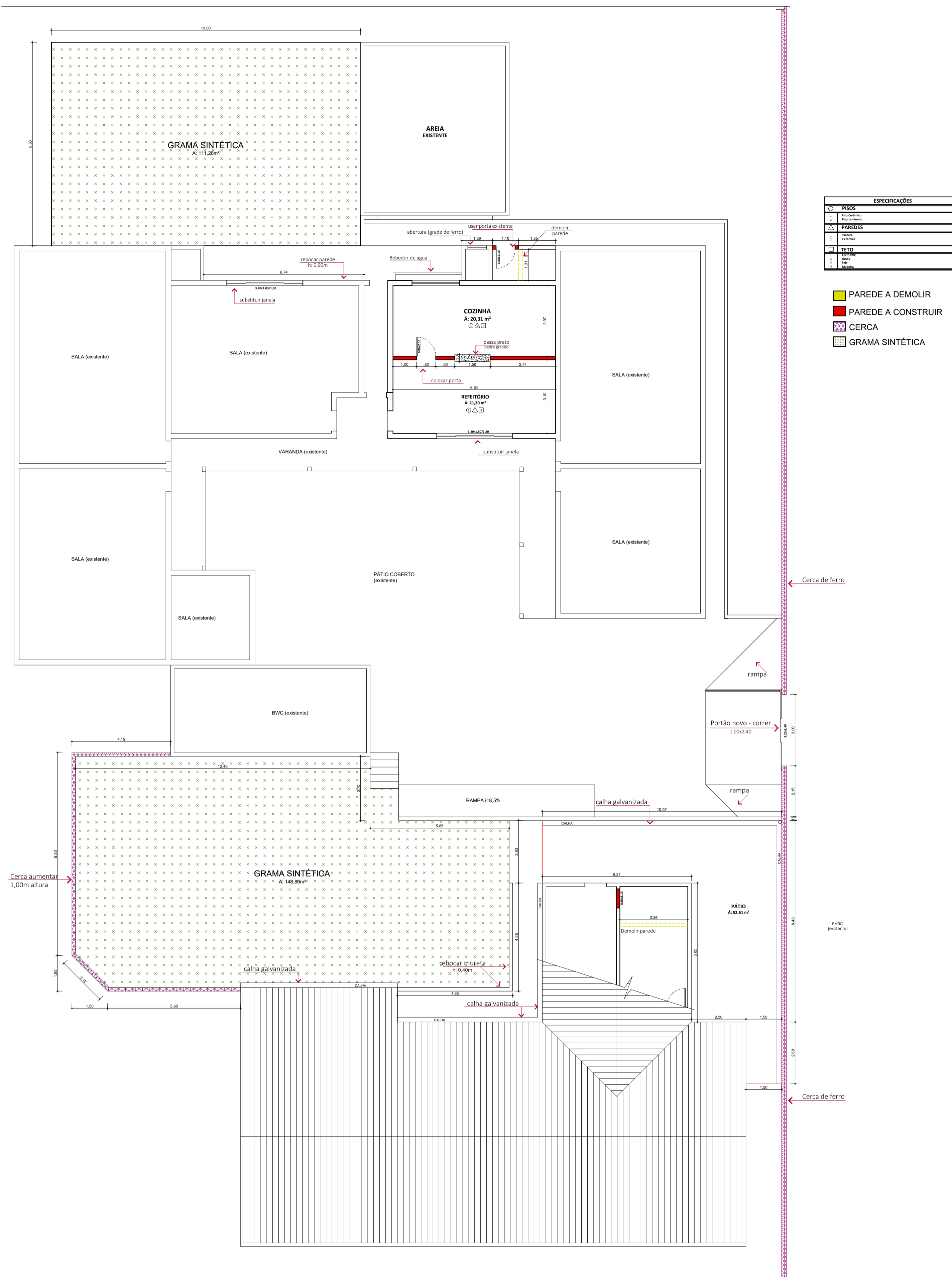
PLANTA BAIXA escala 1/50
