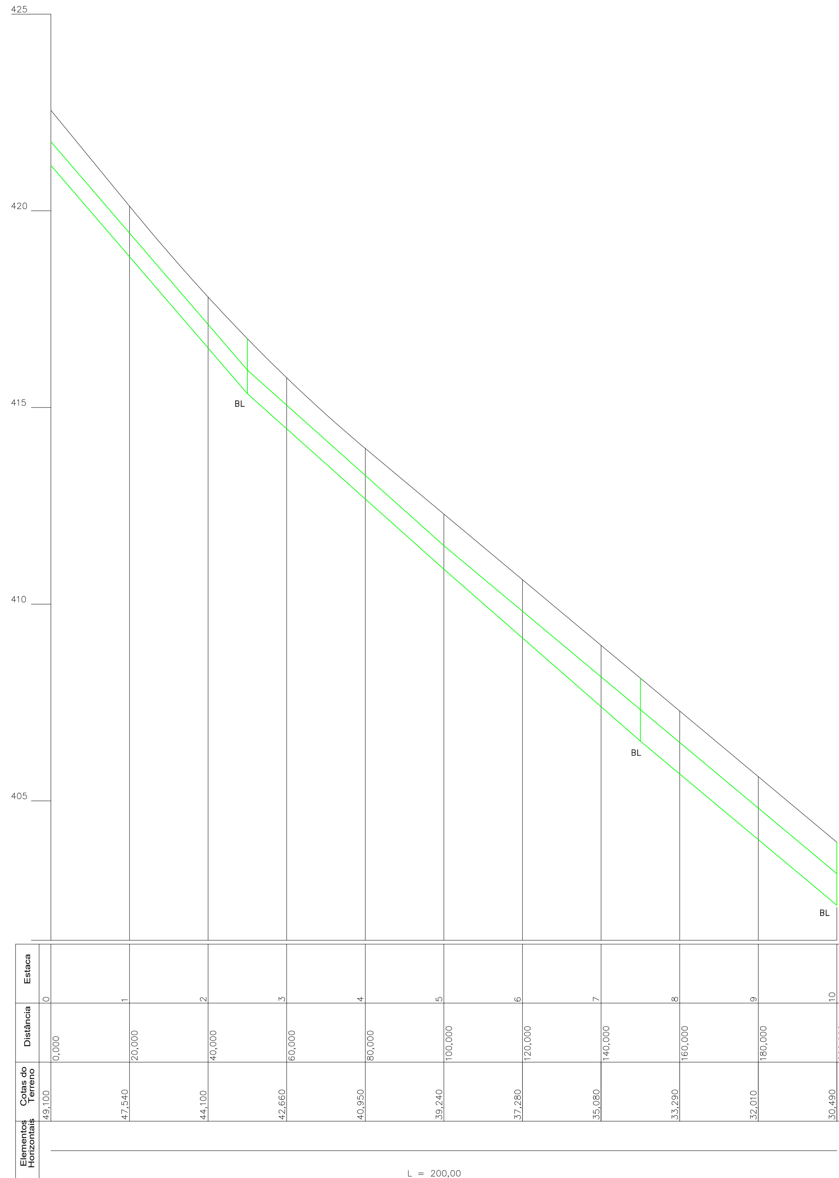
PERFIL LONGITUDINAL – TRAVESSA LUIZ MODESTI Escala: ___ 1:600
