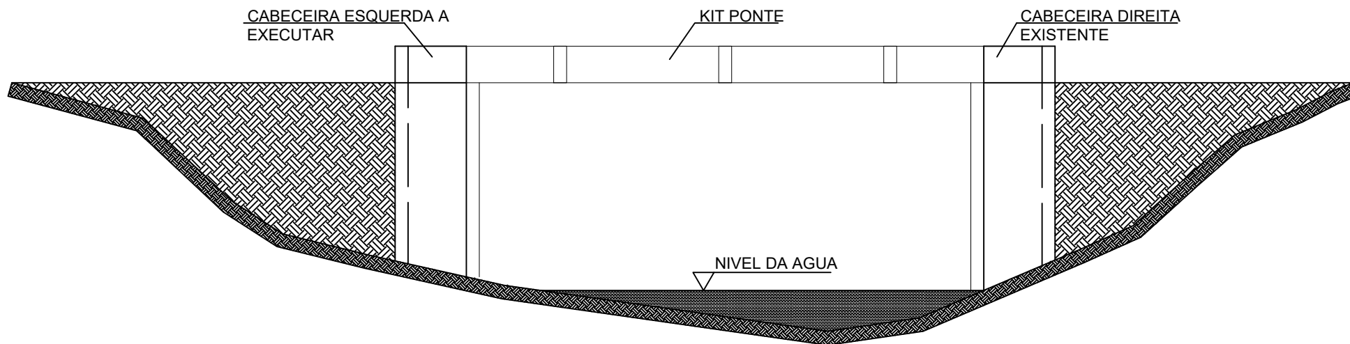
CORTE LONGITUDINAL
