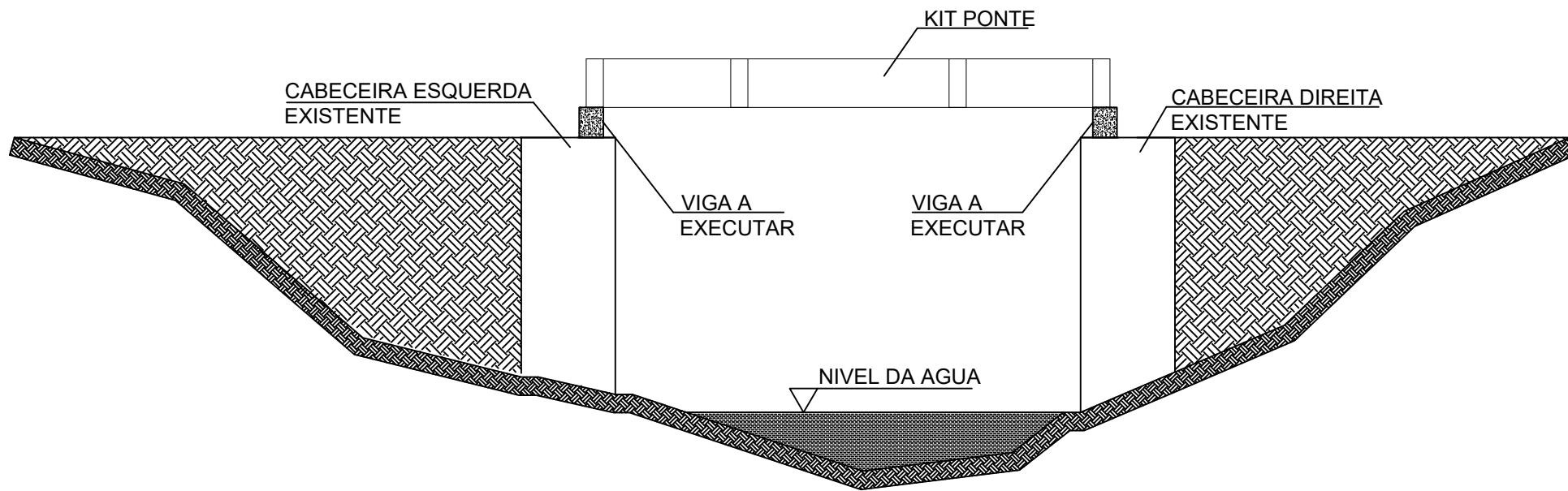
CORTE LONGITUDINAL
