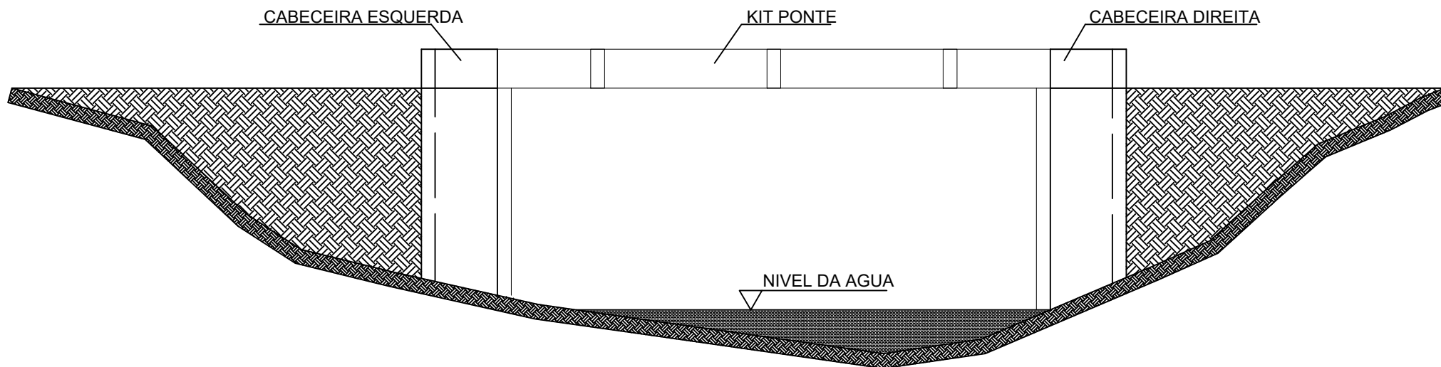
CORTE LONGITUDINAL
