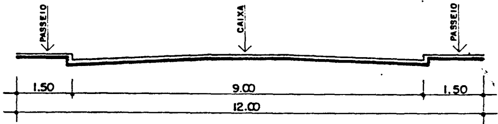
SEÇÃO TRANSVERSAL ESC.: 1: 100
