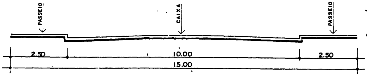
SEÇÃO TRANSVERSAL ESC.: 1: 100
