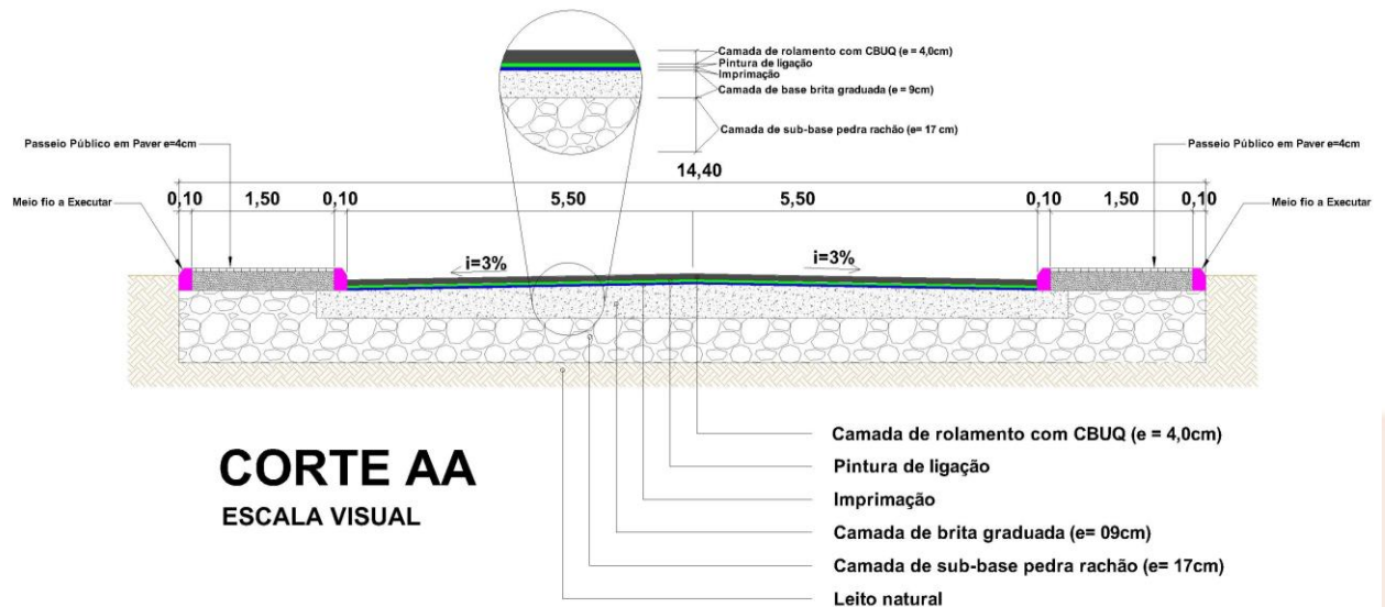
Detalhe 3 – Execução de pavimentação sobre leito natural
