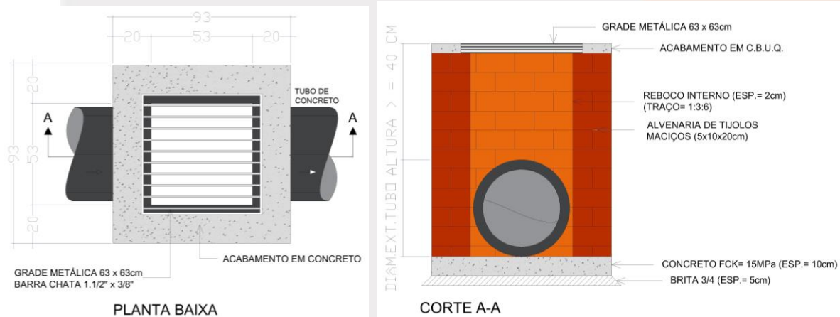
Detalhe 1 – Detalhe Boca de Lobo Ø40cm
