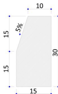
Detalhe 2 – Meio Fio Simples Extrusado
